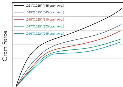
Rectangular SE
