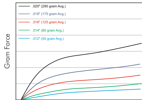
Round SE
